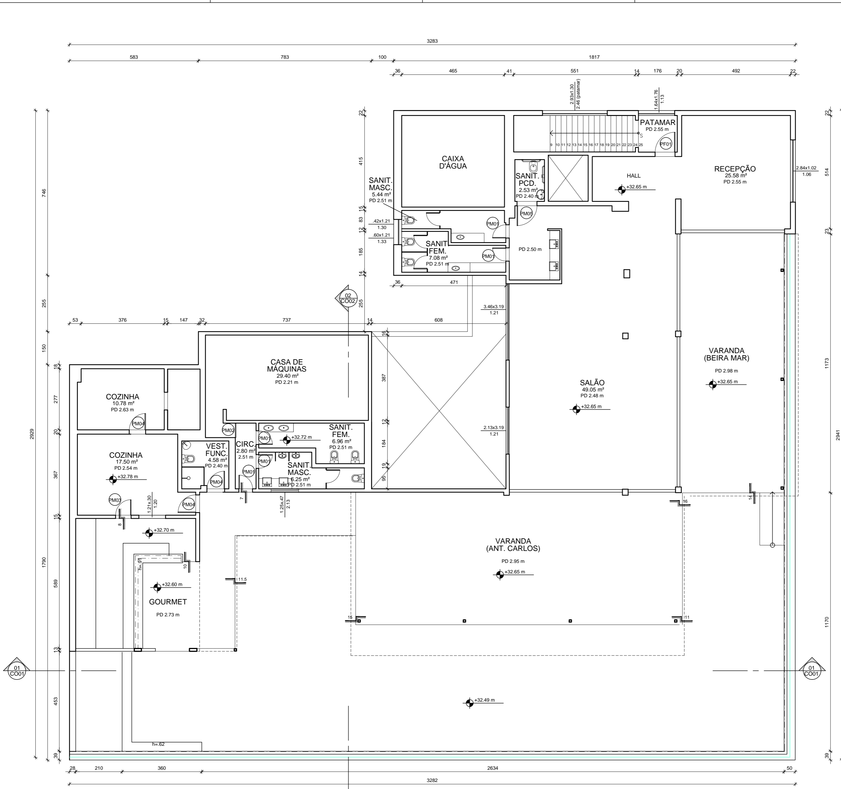
01 PLANTA BAIXA - 9º PAVIMENTO ESC.: 1/100
